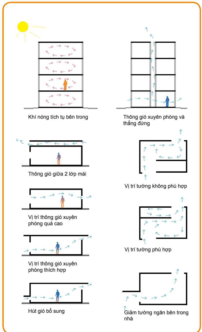
Các dạng kết cấu thông gió tự nhiên (Nguồn: Hesse 2009)
