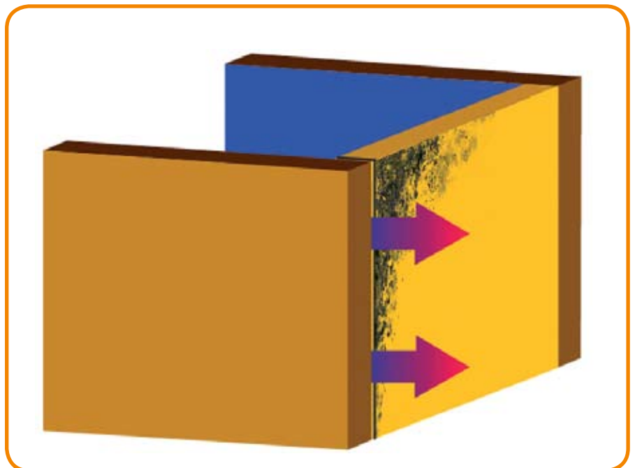
Không khí lọt qua khe tại chỗ nối của tường, khi đối lưu sẽ làm mát bức tường, gây ra nấm mốc có hại và gây hỏng hóc cho công trình (Nguồn: Hesse 2010)
