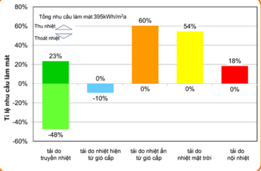
Yêu cầu làm mát của nhà phố điển hình khi sử dụng máy điều hoà (kết quả mô phỏng, Nguồn: Schwede 2009)
