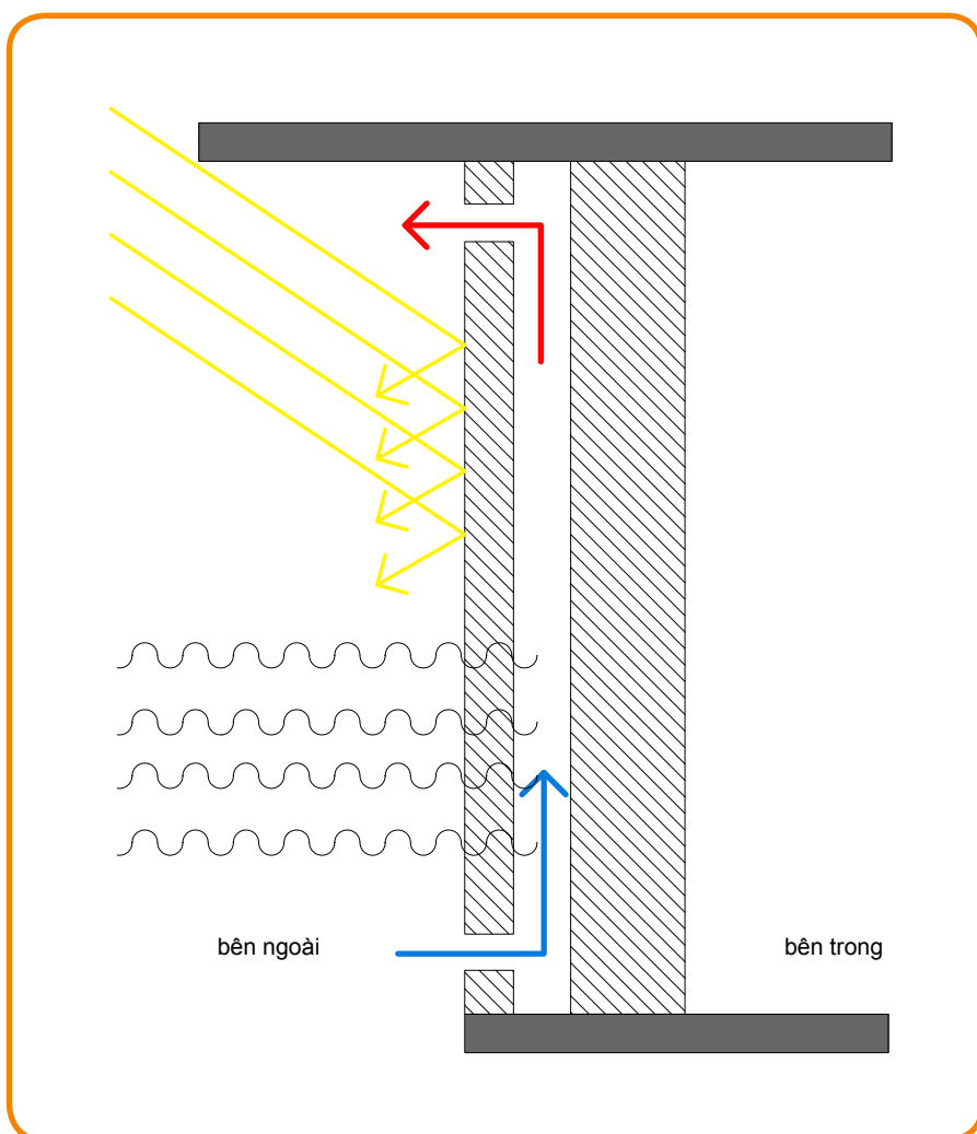
Vỏ bọc công trình 2 lớp có tác dụng chống nắng, thông gió giữ cho nhiệt không vào bên trong ngôi nhà (Nguồn: Hesse 2009)
