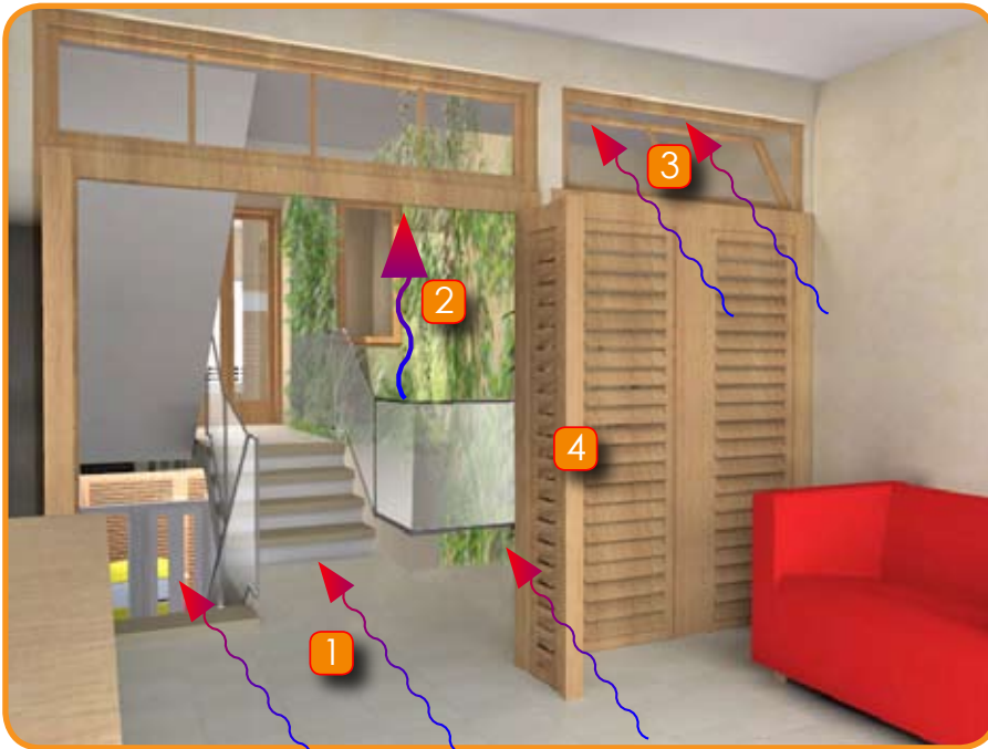
Phương thức thiết kế thông gió bên trong (Nguồn: Hesse 2010)
